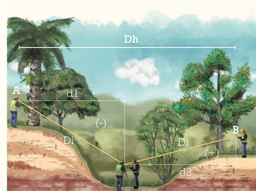
Figura 9. Corrección por pendiente
