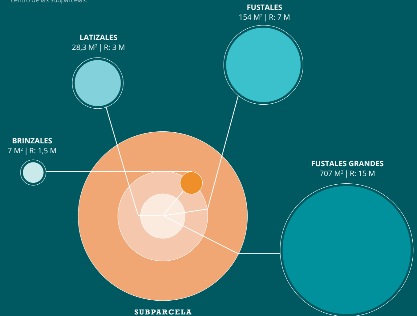
Figura 3. Configuración de subparcela
