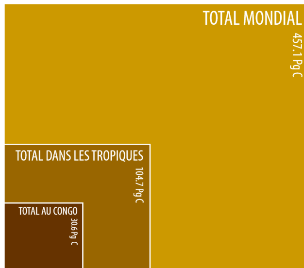
Figure 2. Estimations des réserves de carbone organique dans les tourbières de la Cuvette Centrale du Congo, les tourbières tropicales et mondiales [1-3]
